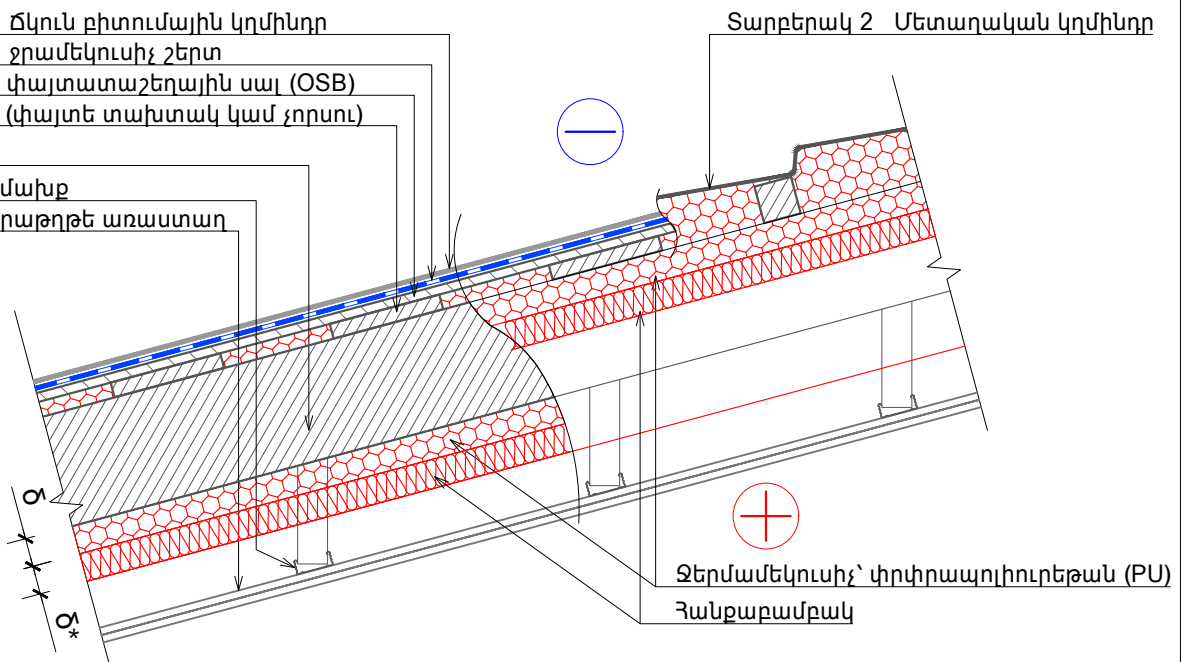
ԿՏՐՎԱԾՔ Ա-Ա
